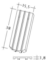
Technický výkres škridla PROFIL Kera-Saechs-15cm-AnAbfuehrer
