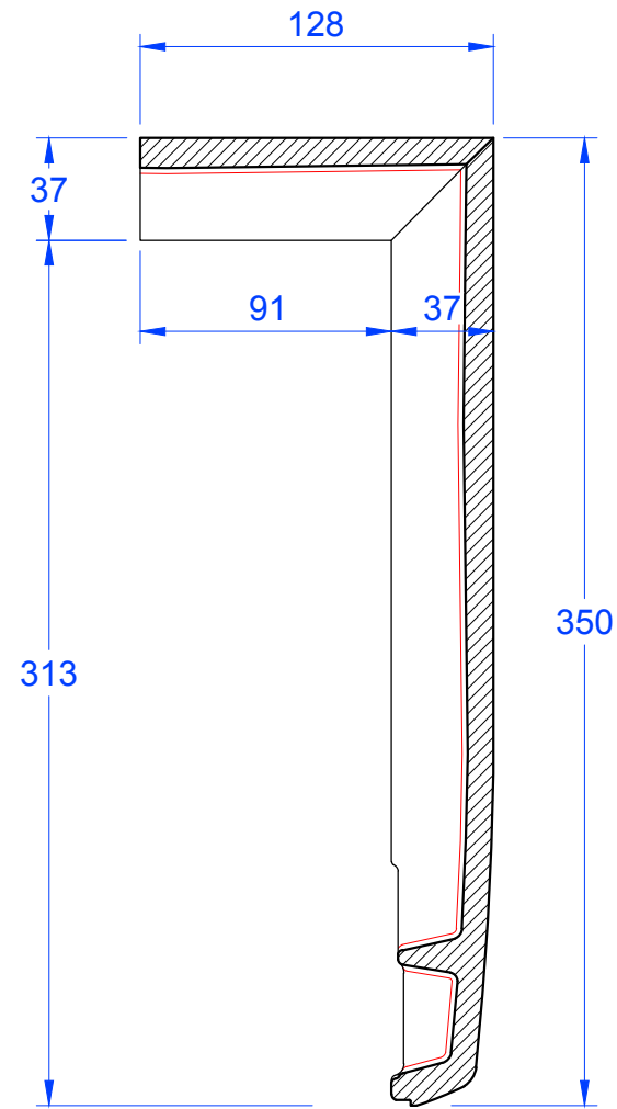
Schnitt B-B
