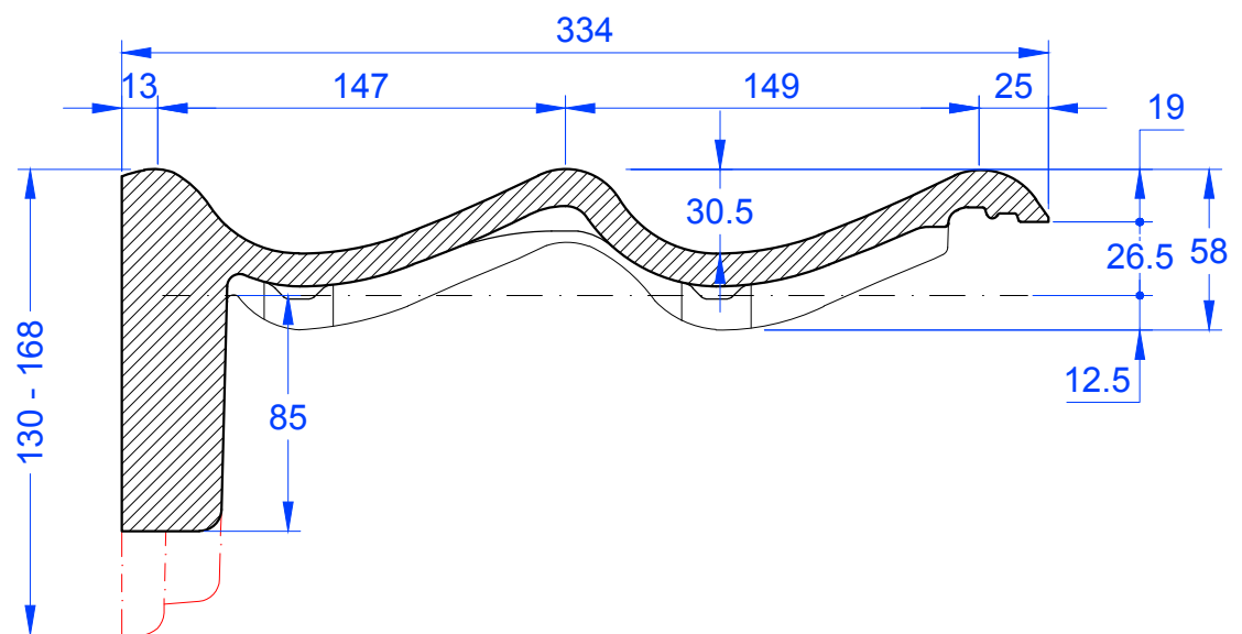
Schnitt A-A
