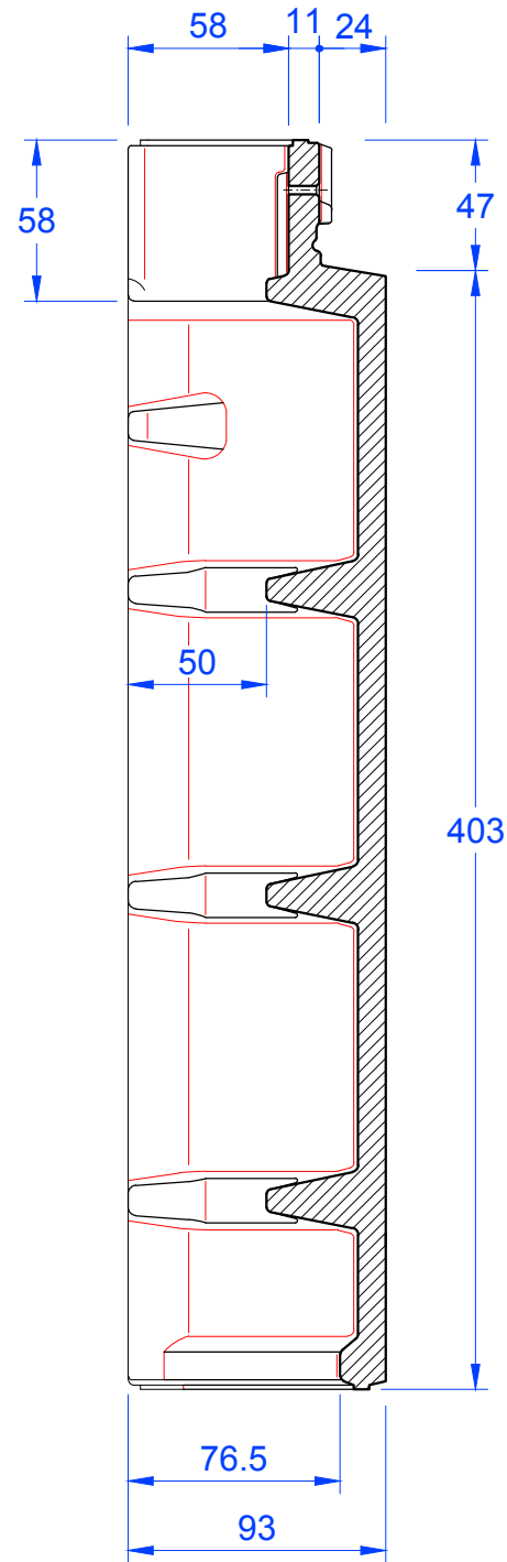
Schnitt A-A
